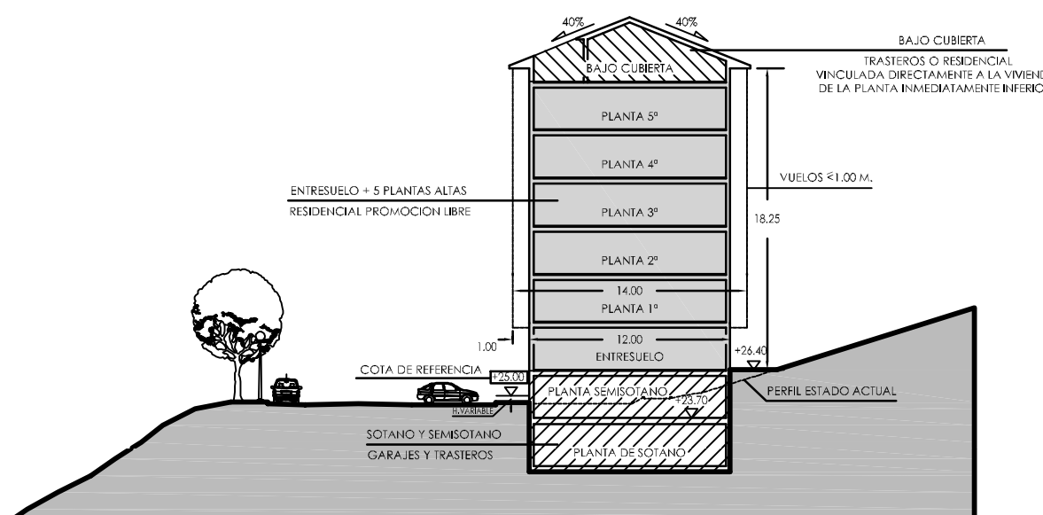
PERFIL A-A
