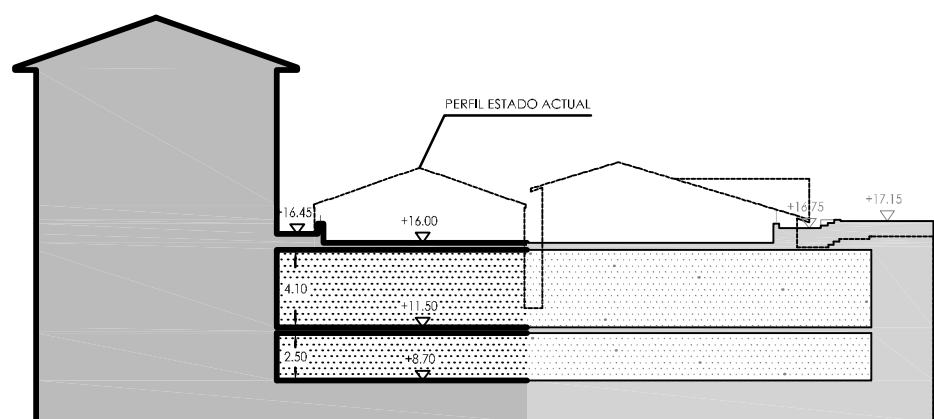
PERFIL A-A
