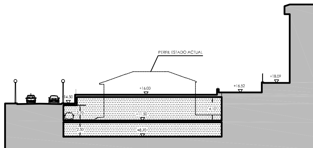
PERFIL C-C
