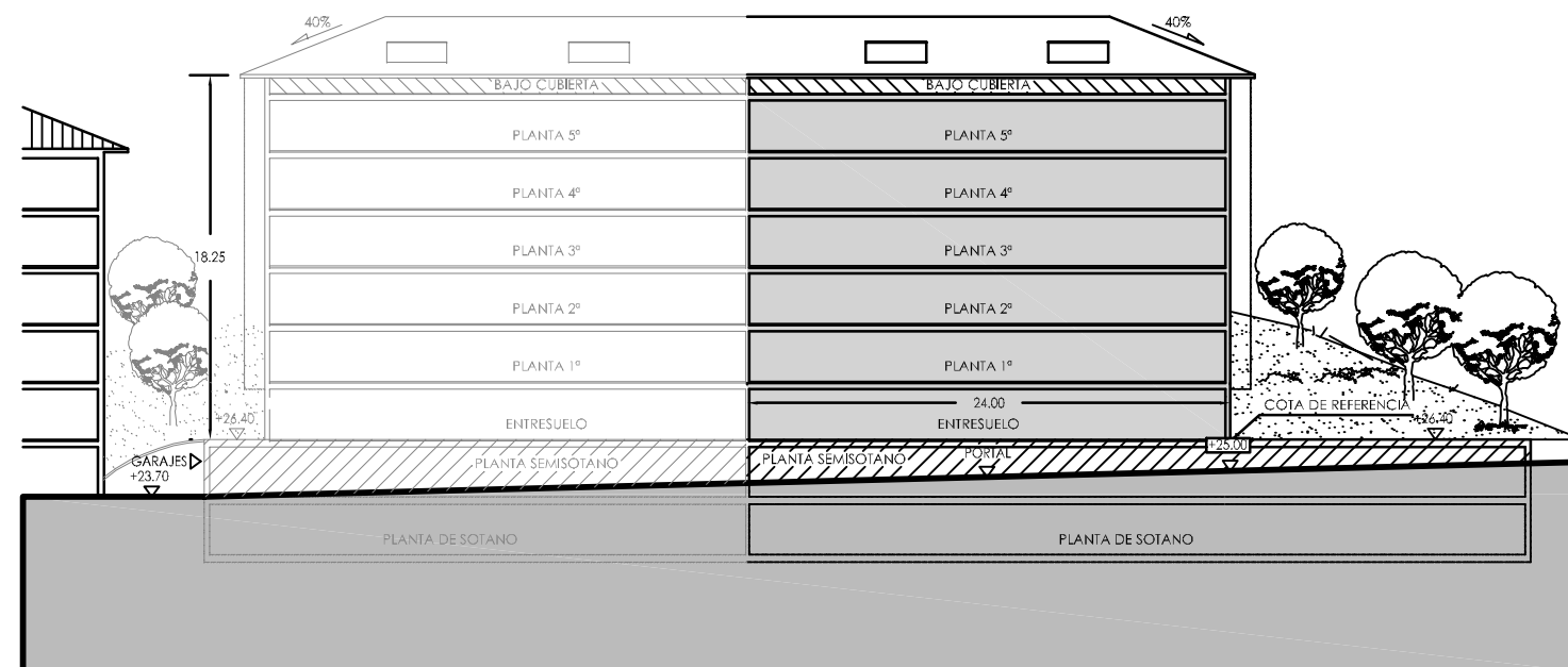
PERFIL B-B
