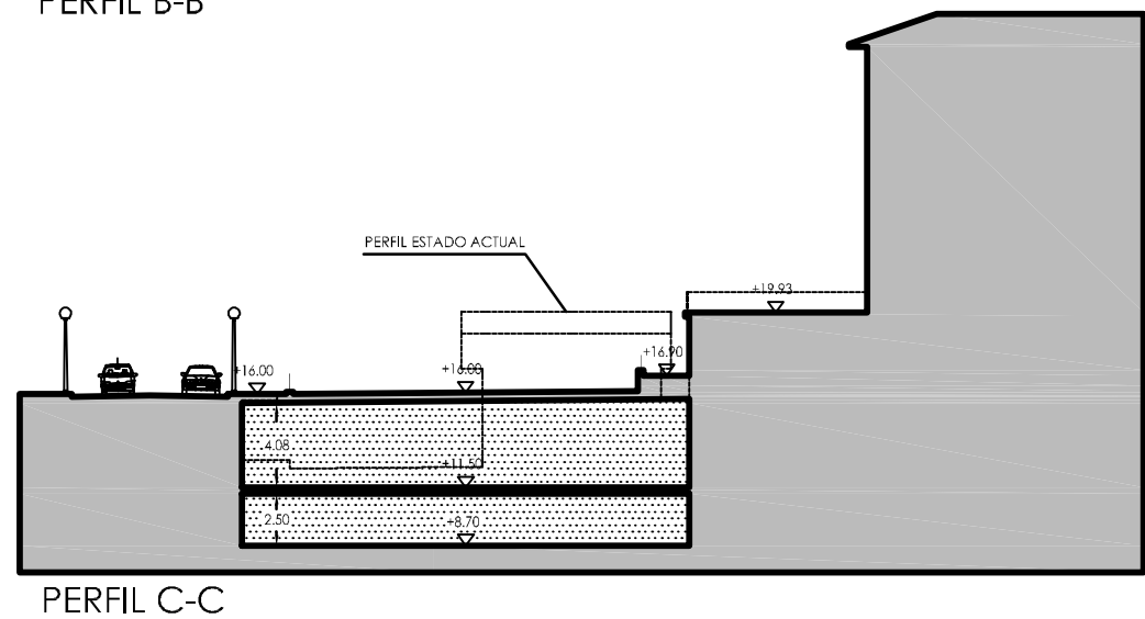
PERFILES LONGITUDINALES Y TRANSVERSALES DE LA ORDENACION PLANTEADA
